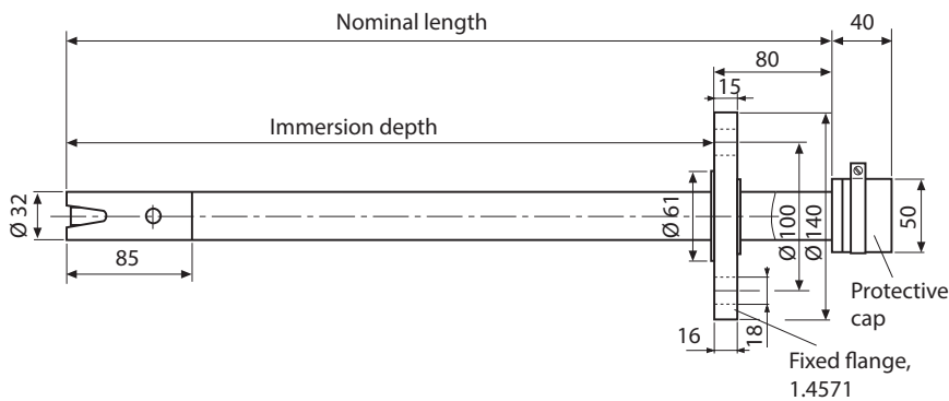
Flange, DN 32 PN 10/16
